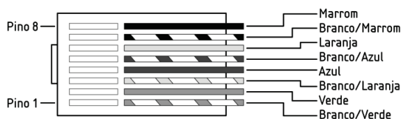
Cabo de rede normal (EIA/TIA-568A)
