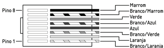
Cabo de rede crossover (EIA/TIA-568B)
